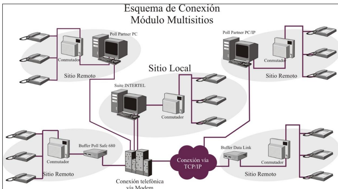
Figura 12.1 Esquema de Conexión Multisitios.
