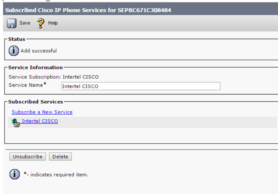
Figura 4.17 Configuración de la aplicación en un teléfono Cisco
