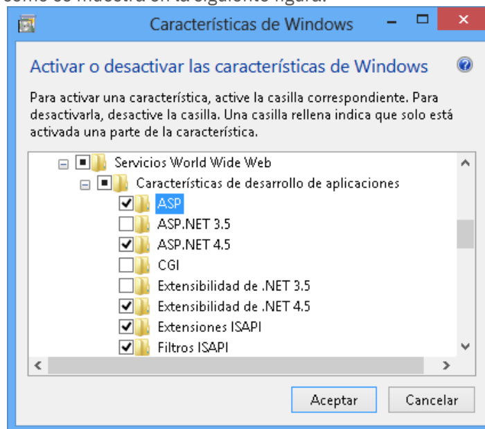
Figura 2.22 Activar servicio ASP y ASP .NET en Windows 8 Profesional o superior
