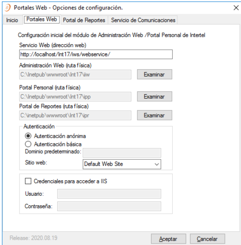
Figura 2.144 Configuración de Portales Web.
