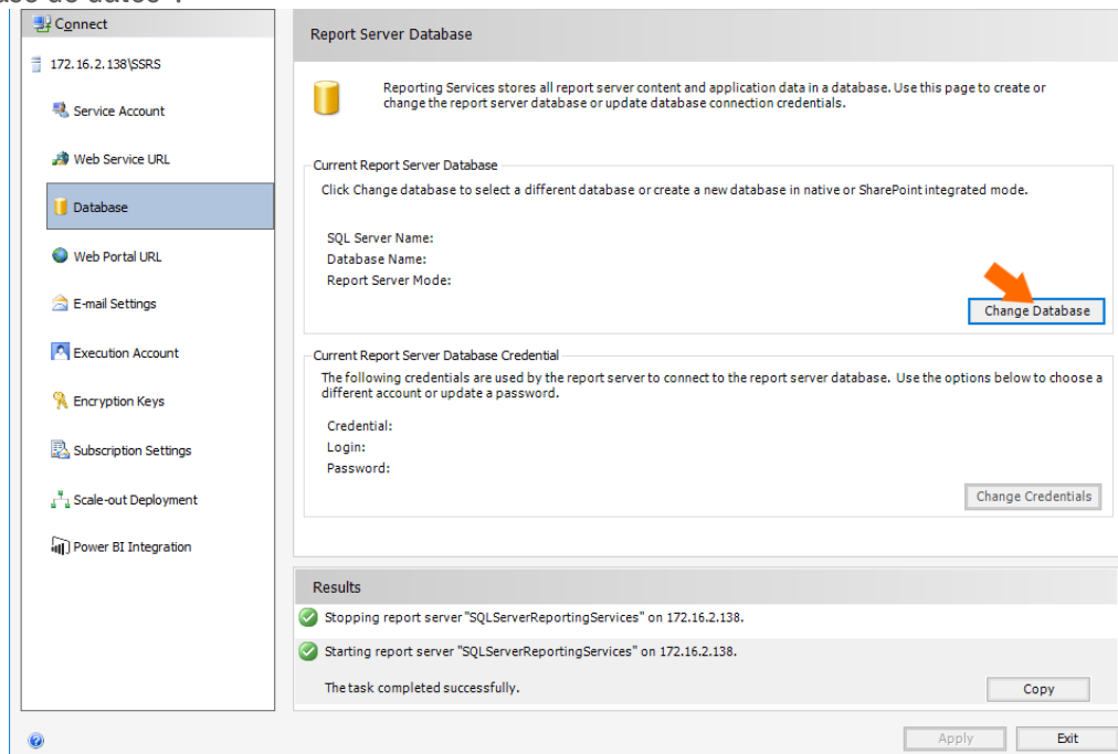
Figura 2.116 Configuración del Servidor SQL de Reporting Services.
