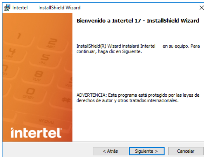
Figura 2.31 Instalando Intertel®
