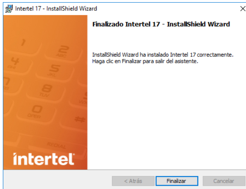
Figura 2.35 Instalando Intertel®
