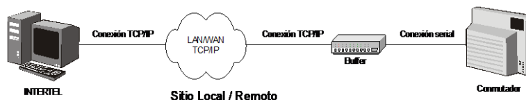
Figura 3.3 Conexión TCP/IP con Buffer Hardware
