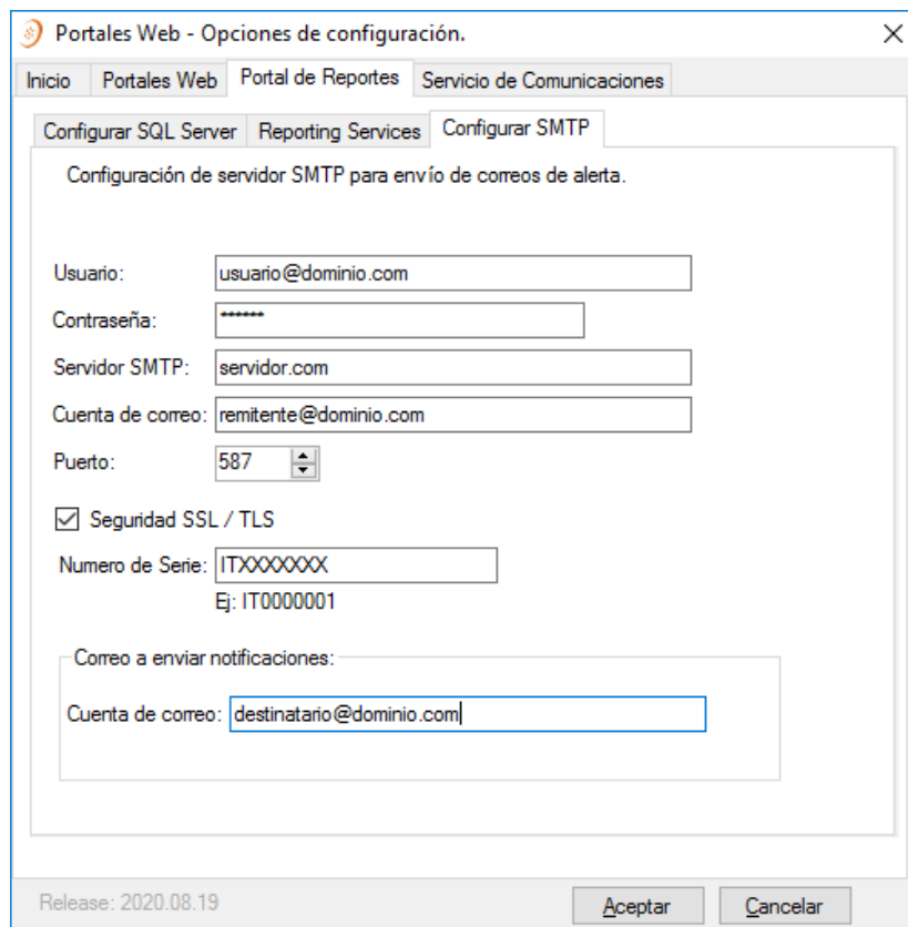
Figura 2.138 Configuración de Portales Web.
