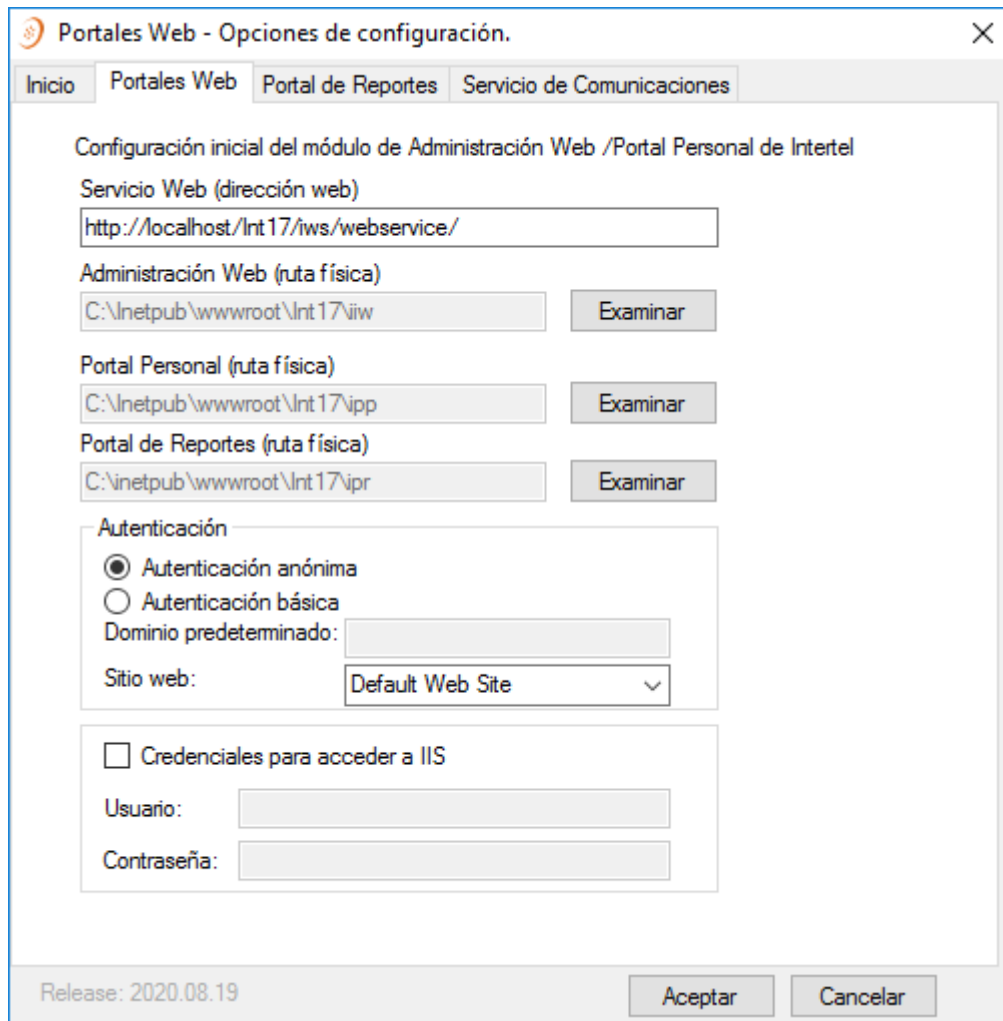
Figura 2.59 Configuración de ruta física del servicio web.
