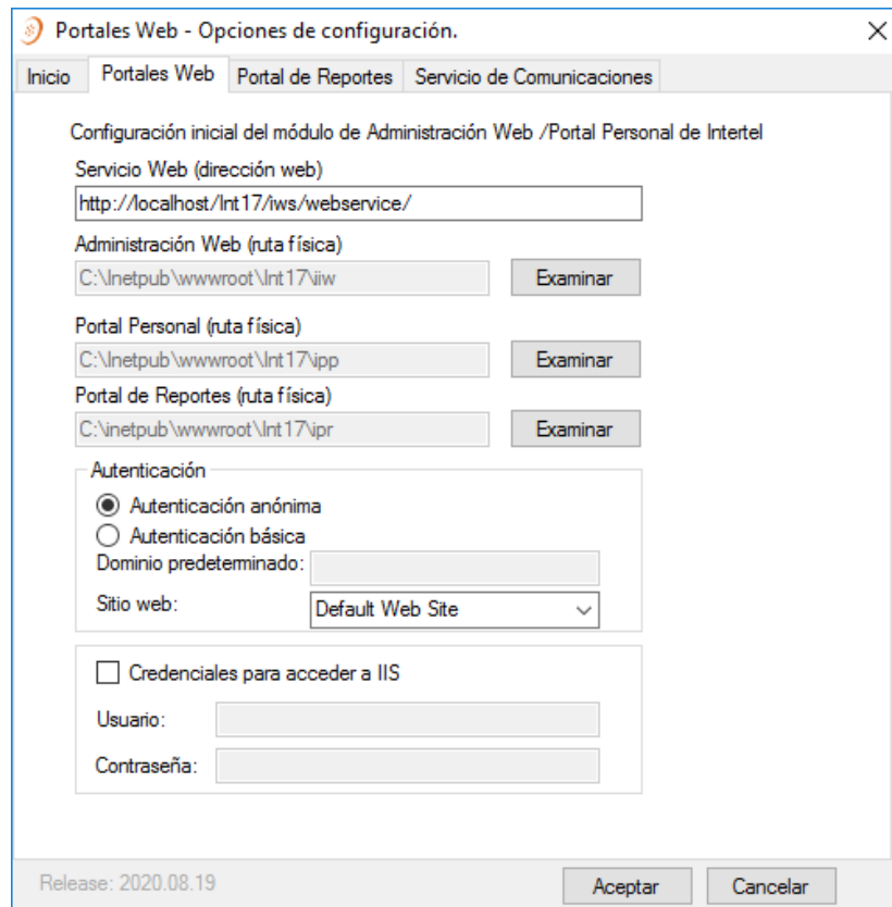
Figura 2.133 Configuración de Portales Web.
