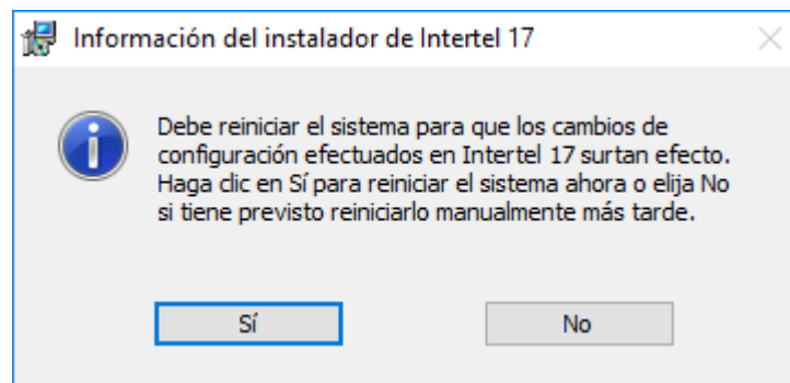
Figura 2.36 Instalando Intertel®
