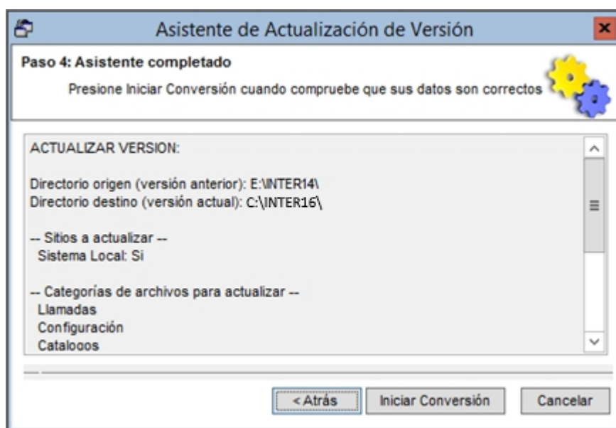
Figura C.4 Asistente completado
