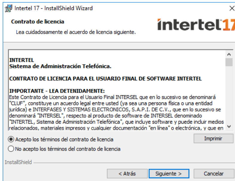
Figura 2.32 Instalando Intertel®
