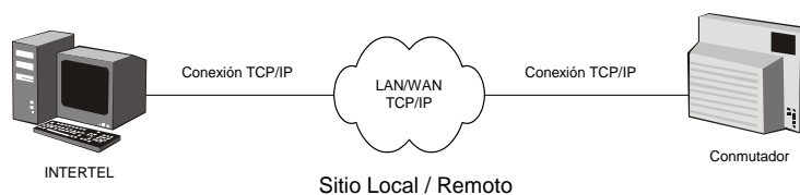
Figura 15.3 Conexión TCP/IP.
